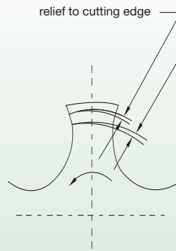
Eccentric Relief
